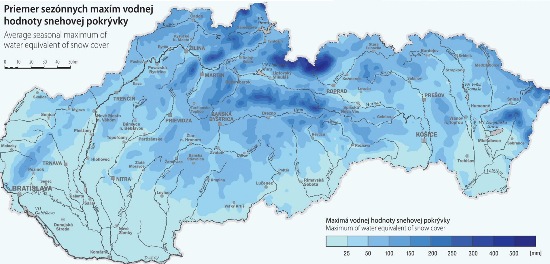
Maximálna vodná hodnota snehovej pokrývky Maximum of water equivalent of snow cover
