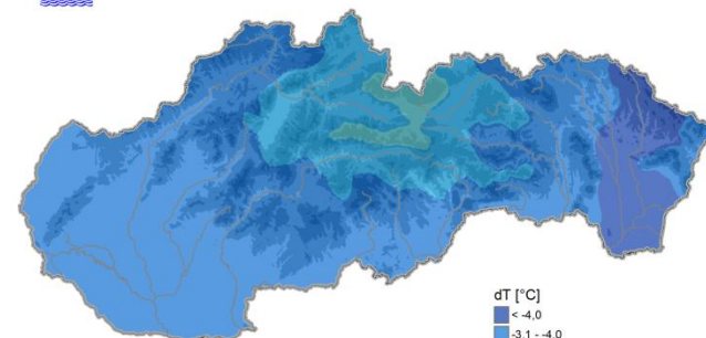
Odchýlka priemernej teploty vzduchu za zimu 1963/64 od normálu 1961-1990
