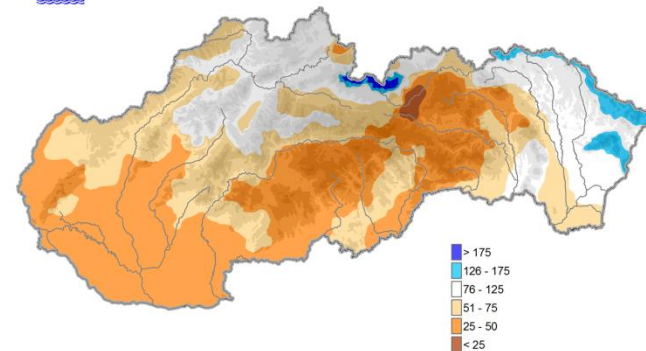
Úhrny atmosférických zrážok za zimu 2016/17 v % normálu 1961-1990
